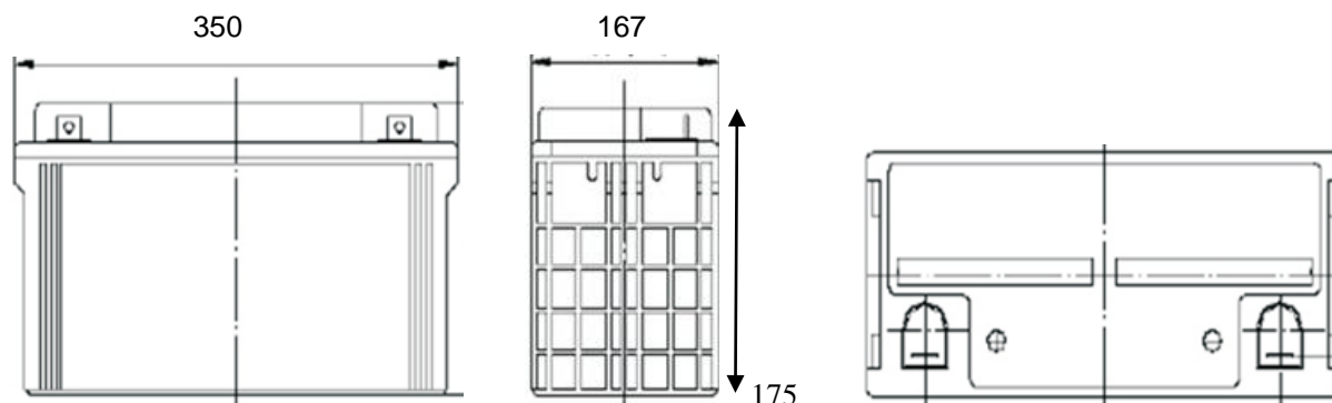
Габаритные размеры и расположение клемм АКБ
