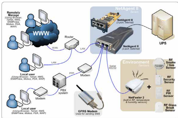
Рис.1 Подключение NetFeeler 2
