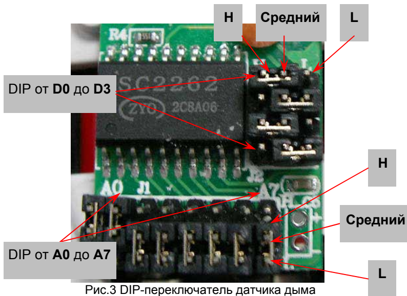
Рис.3 DIP-переключатель датчика дыма
